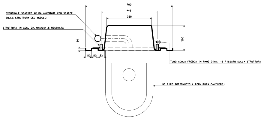
PIANTA
