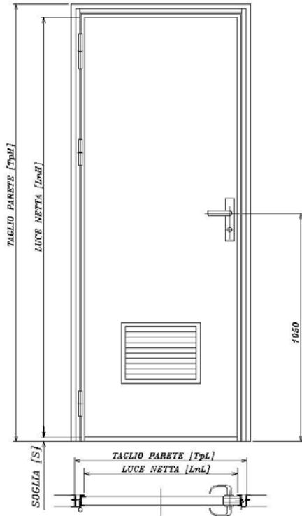
PORTA CON TELAIO A "T" VISTA INTERNA - LATO CERNIERE
